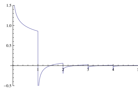
(h) \alpha = 0.8
