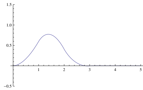
(d) \alpha = 3.2
